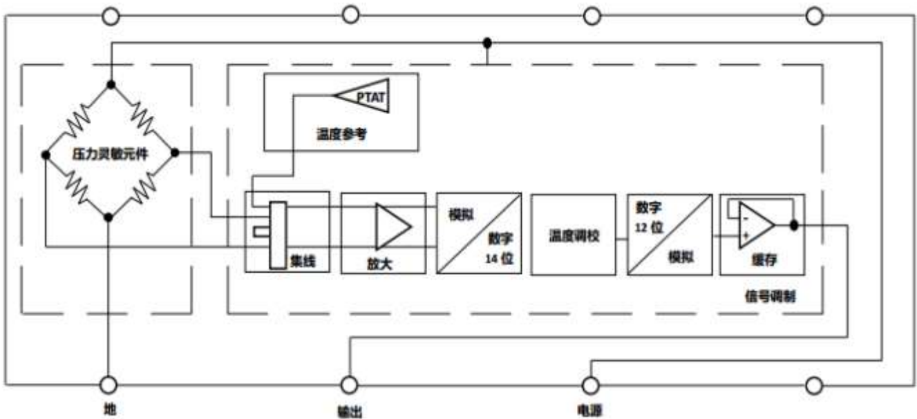
LW181 模拟放大输出等效电路
