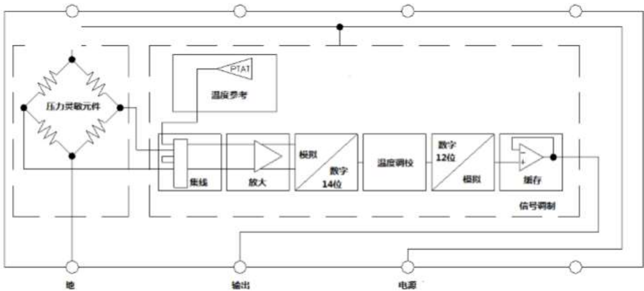
LW55 模拟放大输出等效电路
