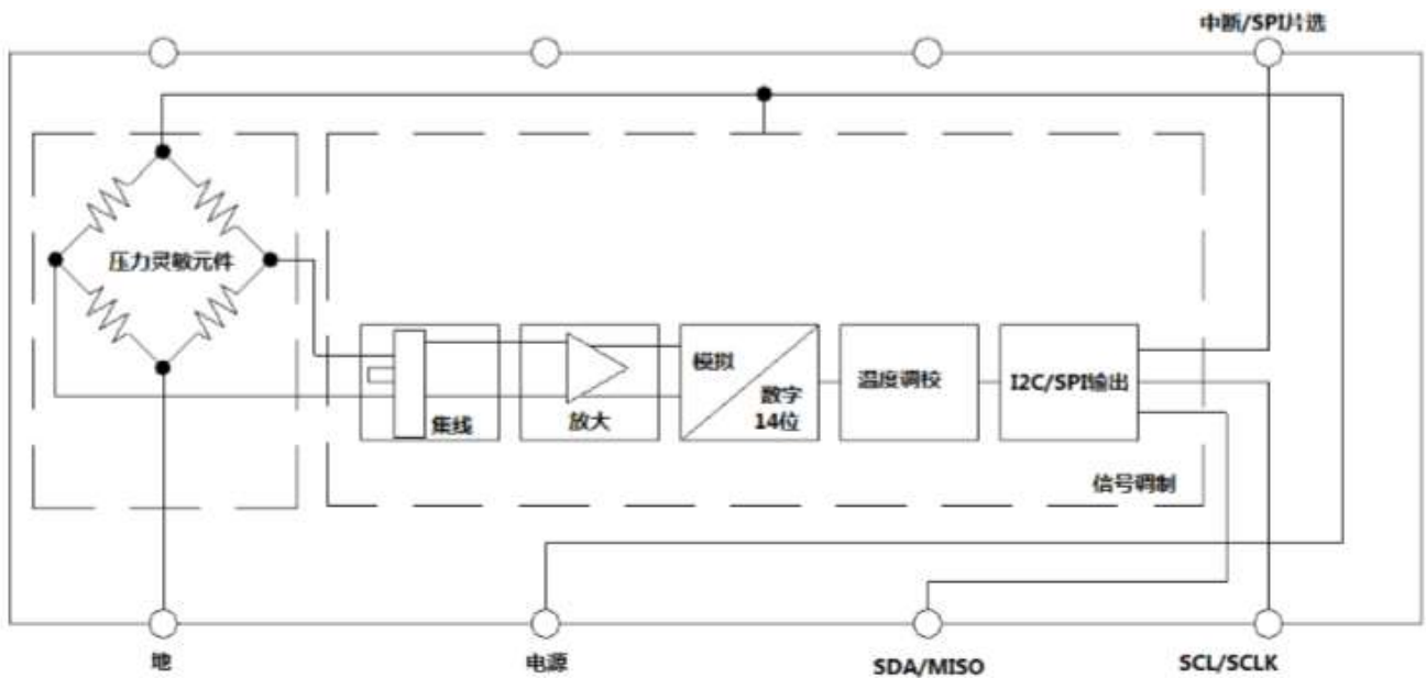
LW56 数字输出等效电路
