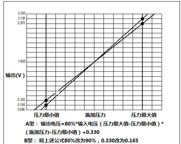
压力转换方程, 电压输入3.3V
